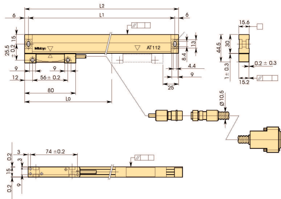
L0 Efektywny zakres pomiaru L1 Rozstaw otworów montażowych L2 Długość całkowita
