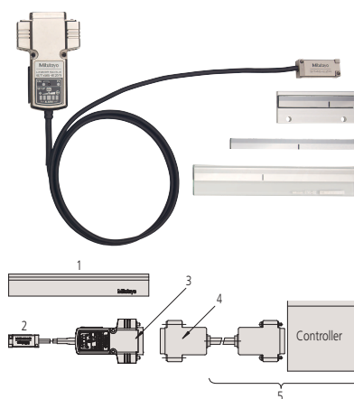
1: Liniał - element główny; 2: Detektor; 3: Złącze sygnałowe (w zestawie); 4: Kabel sprężenia zwrotnego; 5: Do doposażenia przez klienta (kabel/sterownik sprężenia zwrotnego)
