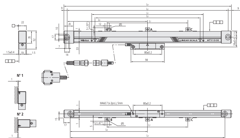
Sposób montażu Nr1-Nr2
